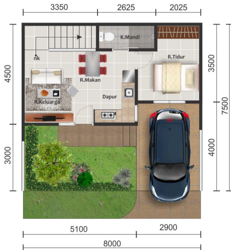
Denah Lt. Dasar
