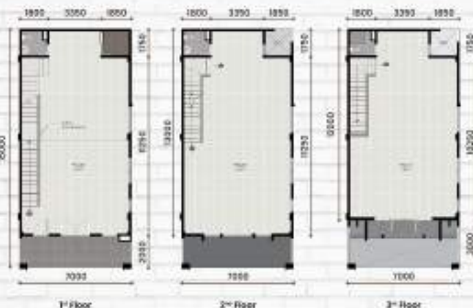
Hoek Type 7 x 15 LT : 105 m 2 | LB : 268 m 2
