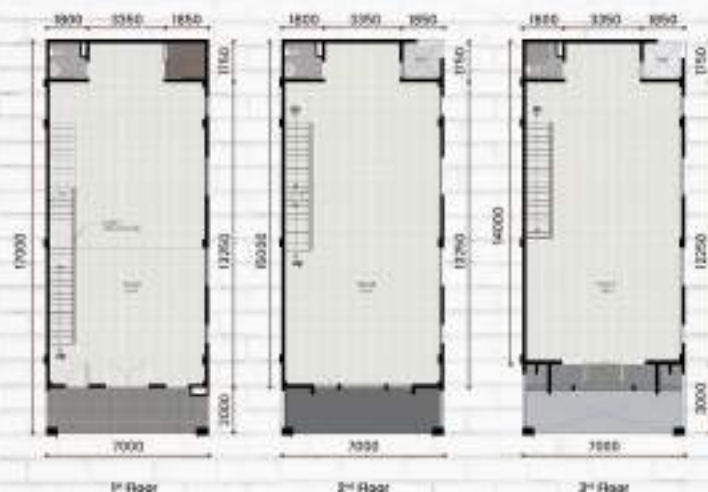
Hoek Type 7 x 17 LT : 119 m 2 | LB : 310 m 2
