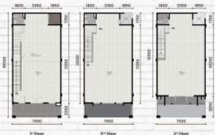
Standard Type 7 x 15 LT : 105 m 2 | LB : 268 m 2
