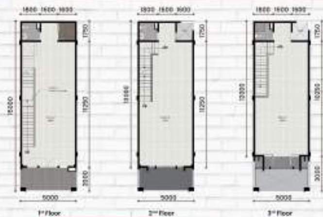
Standard Type 5 x 15 LT : 75 m 2 | LB : 190 m 2
