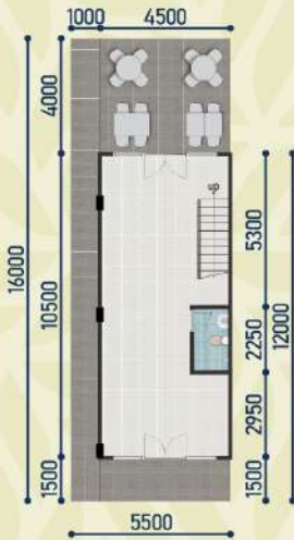
Lantai Dasar
