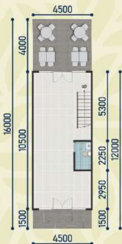
Lantai Dasar
