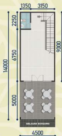
Lantai Dasar
