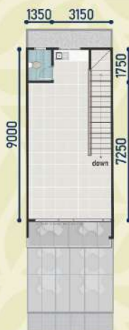
Lantai 3
