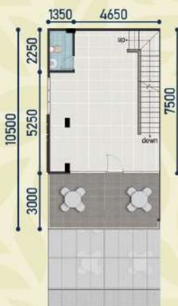
Lantai 2
