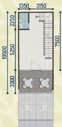
Lantai 2
