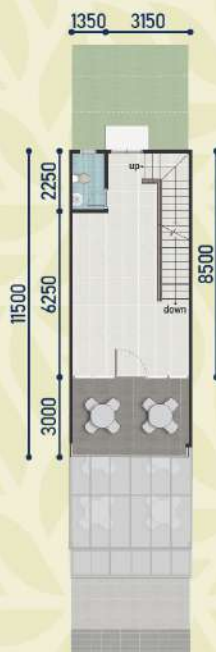
Lantai 2
