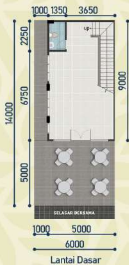
Lantai Dasar
