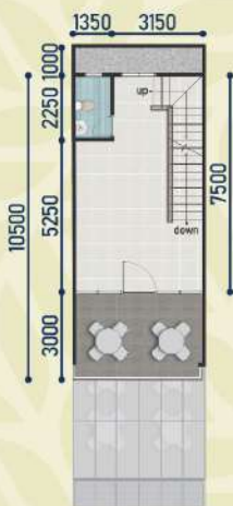
Lantai 2
